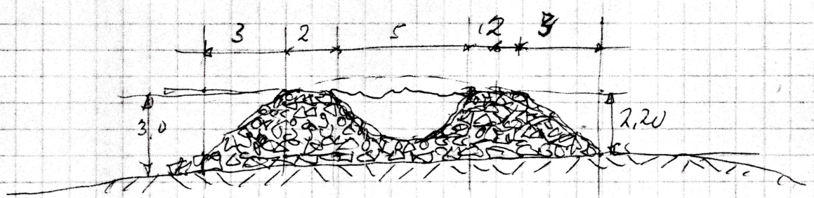
Snitt B-B
