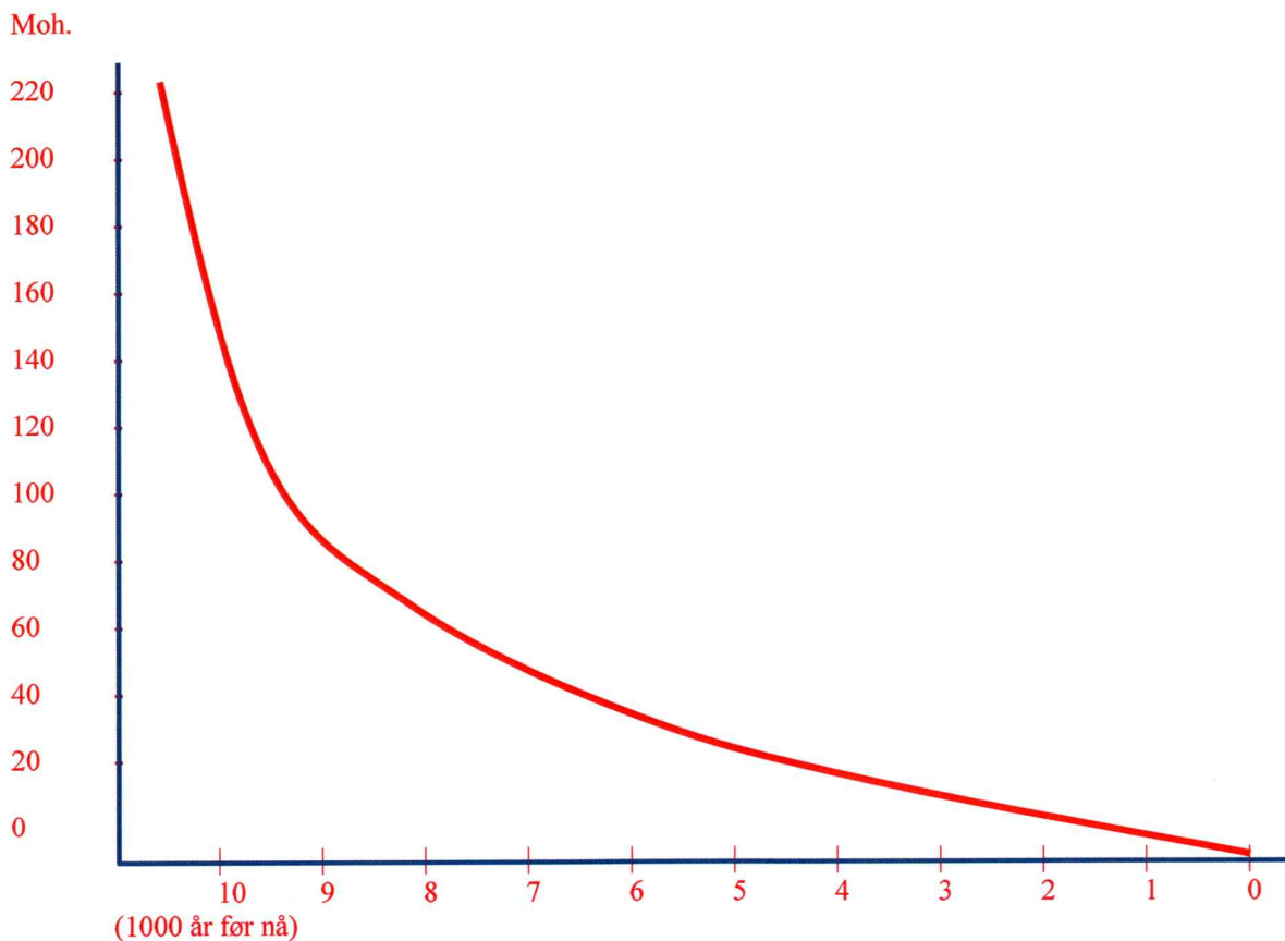
Landhevingsskurve fra Skimorenen. Etter Sørensen 1979.
