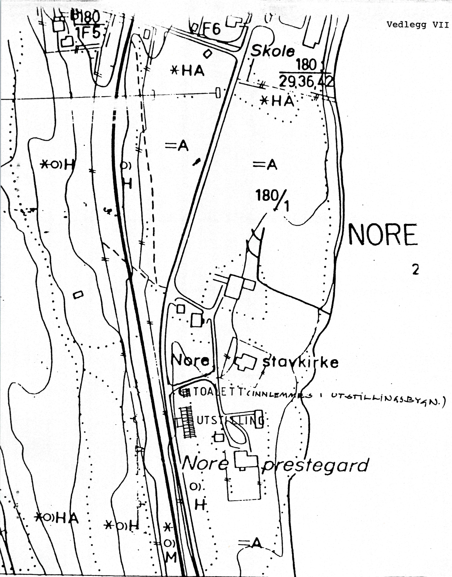
SKISSE UTSTILLINGSBYGNING VED NORE PRESTEGÅRD. MÅL 1:2000
